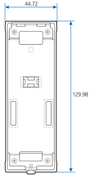
拡張ブラケット
