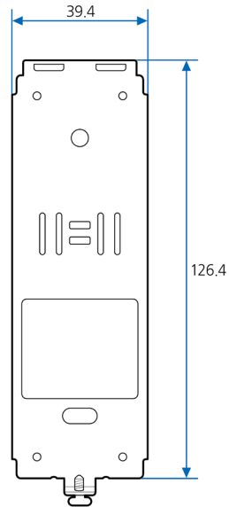
メインブラケット
